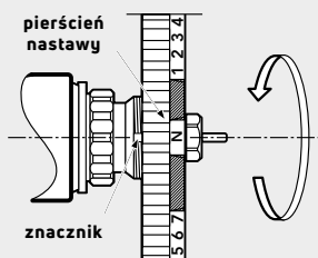
szczegóły „X”
