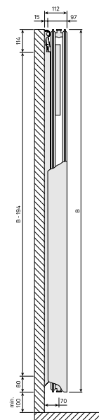
DimensionalDrawing - Tinos V / Paros V, tipas 21, vaizdas iš šono
