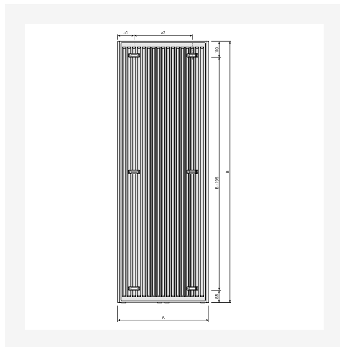
DimensionalDrawing - Tinos V, tipas 21, vaizdas iš galo
