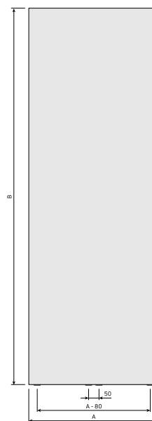
DimensionalDrawing - Tinos V, vaizdas iš priekio
