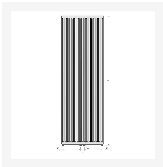
DimensionalDrawing - Vertical, tüüp 10, eestvaade
