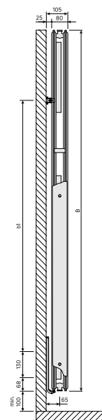
DimensionalDrawing - Vertical, tüüp 21, külgsaade
