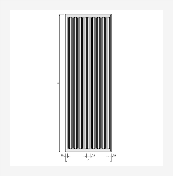
DimensionalDrawing - Vertical, tüübid 20, 21, 22, eestvaade
