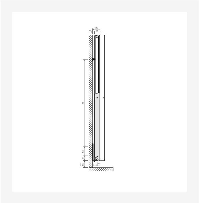
DimensionalDrawing - Vertical, tüüp 20, külgaade
