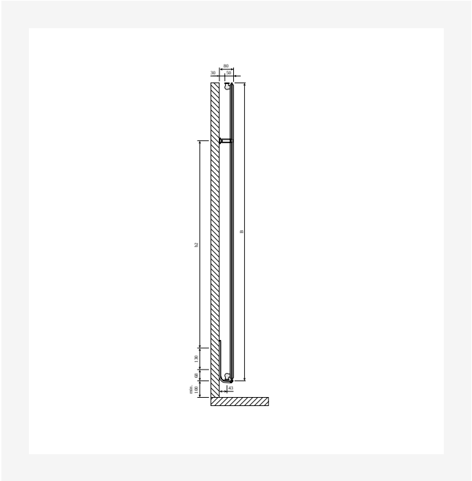
DimensionalDrawing - Vertical, tüüp 10, külgaade
