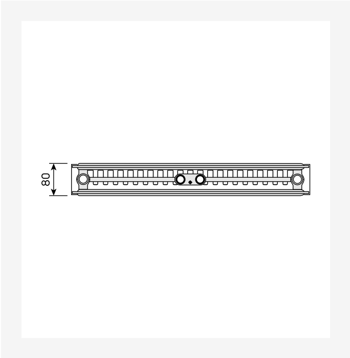
DimensionalDrawing - Vertical, tüüp 21, pealtvaade
