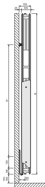
DimensionalDrawing - Vertical, tüüp 22, külgsaade
