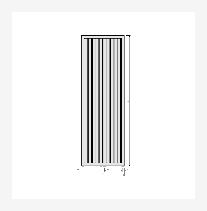
DimensionalDrawing - Vertical, tüüp 10, eestvaade – ilma külgakateteta
