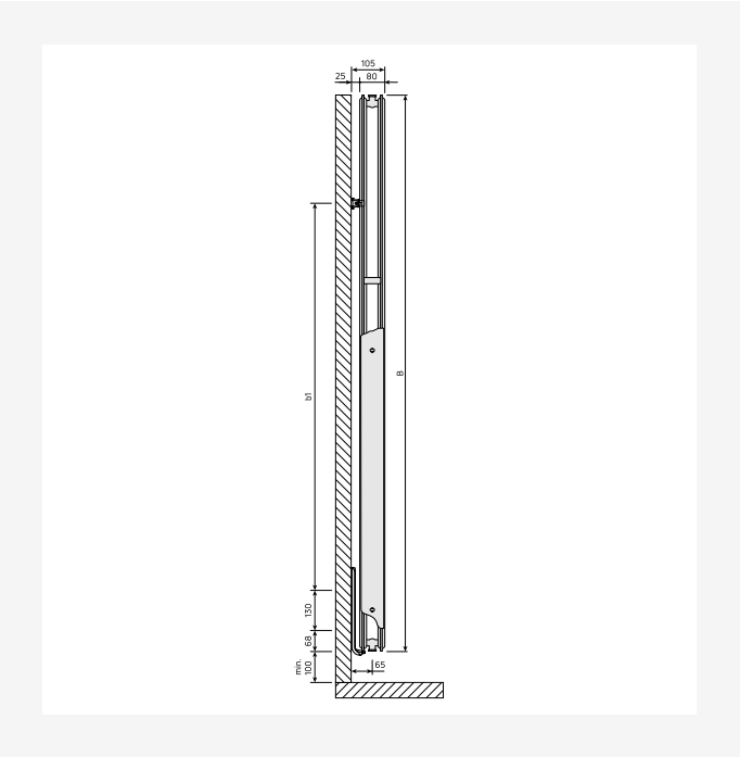
DimensionalDrawing - Vertical, tüüp 20, külgvaade
