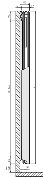
DimensionalDrawing - Tinos V / Paros V, tüüp 21, külgvaade
