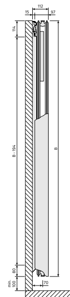
DimensionalDrawing - Tinos V / Paros V, tüüp 21, külgvaade
