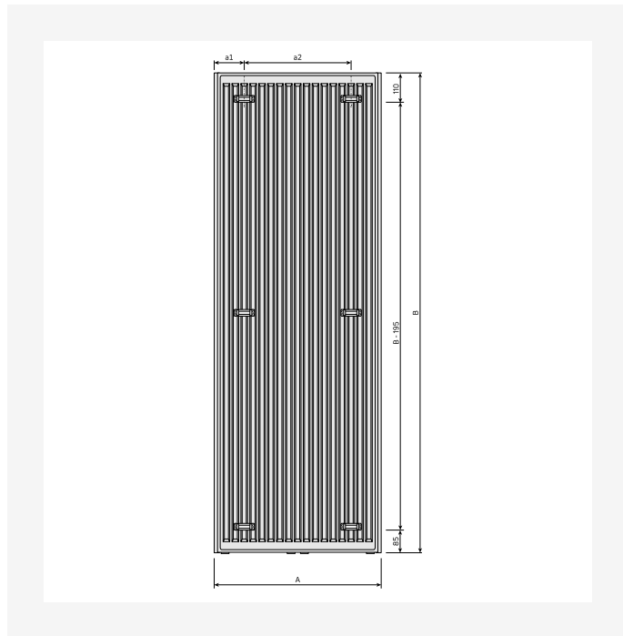
DimensionalDrawing - Tinos V, tüüp 21, tagantvaade
