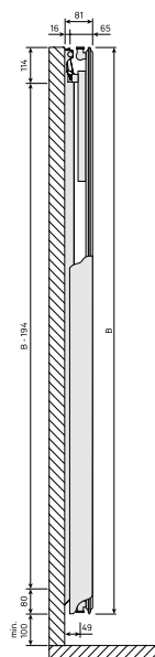
DimensionalDrawing - Tinos V / Paros V, tüüp 11, külgvaade
