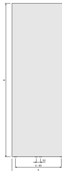
DimensionalDrawing - Tinos V, eestvaade
