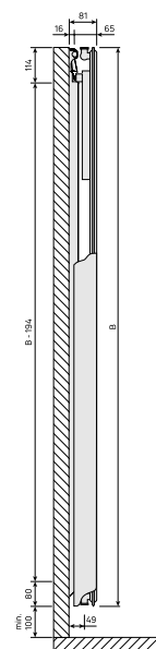
DimensionalDrawing - Tinos V / Paros V, tüüp 11, külgsaade
