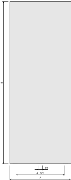
DimensionalDrawing - Paros V, tüüp 11, eestvaade
