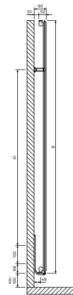
DimensionalDrawing - Vertical, tipas 10, vaizdas iš šono
