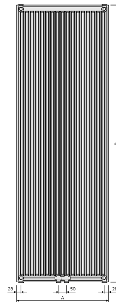
DimensionalDrawing - New Vertical, vaizdas iš galo
