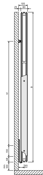
DimensionalDrawing - Vertical, tipas 20, vaizdas iš šono
