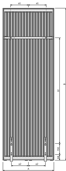
DimensionalDrawing - Vertical, tipai 20, 21, 22, vaizdas iš galo
