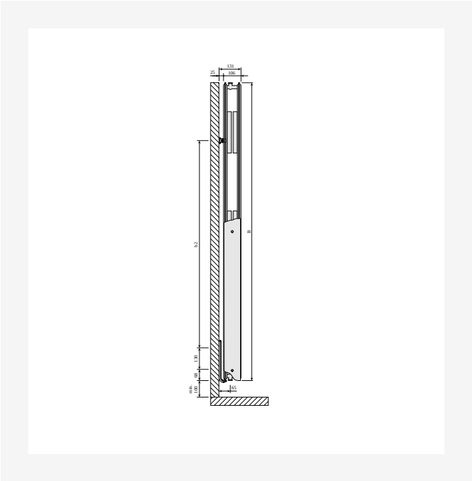
DimensionalDrawing - Vertical, tipas 22, vaizdas iš šono
