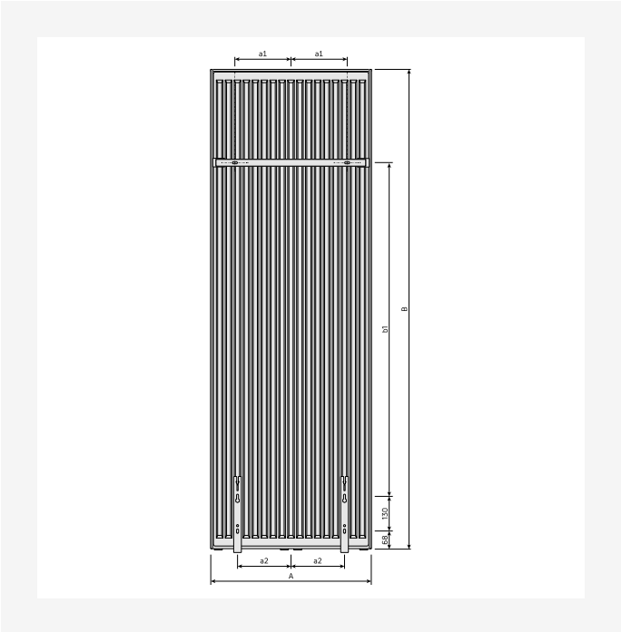
DimensionalDrawing - Vertical, tipai 20, 21, 22, vaizdas iš galo
