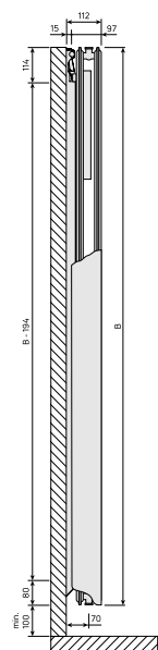
DimensionalDrawing - Tinos V / Paros V, tipas 21, vaizdas iš šono
