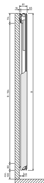
DimensionalDrawing - Tinos V / Paros V, tipas 11, vaizdas iš šono
