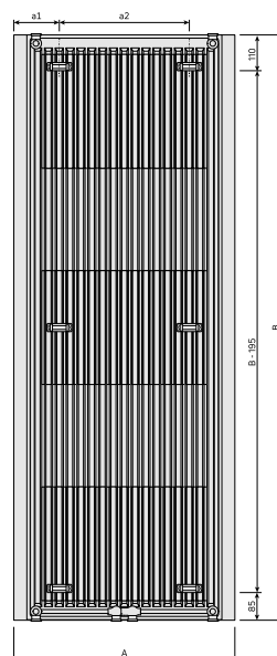
DimensionalDrawing - Paros V, tipas 11, vaizdas iš galo
