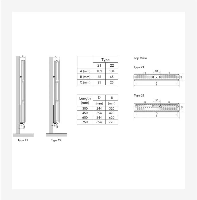
DimensionalDrawing - Purmo Plan & Plan Plus Vertical – montavimo padėty's ir matmenys
