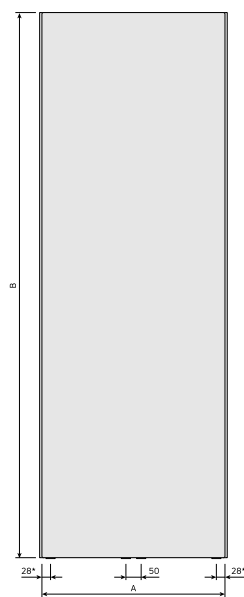
DimensionalDrawing - Kos V, vaizdas iš priekio
