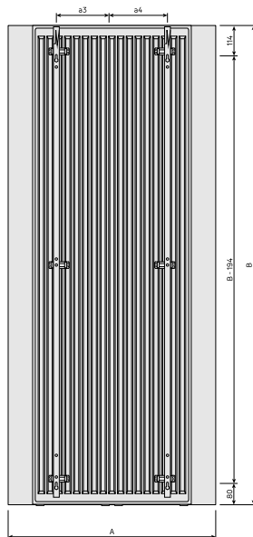
DimensionalDrawing - Paros V, tips 21, skats no aizmugures ar MCWV kronšteinu
