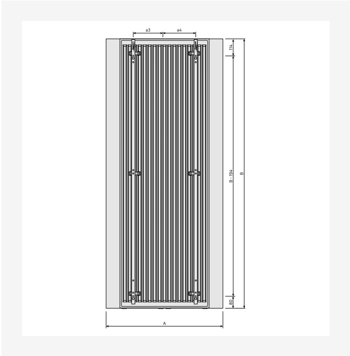
DimensionalDrawing - Paros V, tips 21, skats no aizmugures ar MCWV kronšteinu
