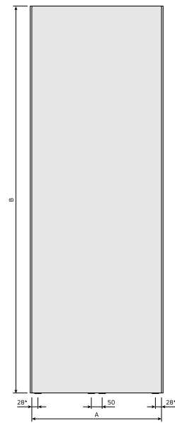
DimensionalDrawing - Kos V, skats no priekšpuses
