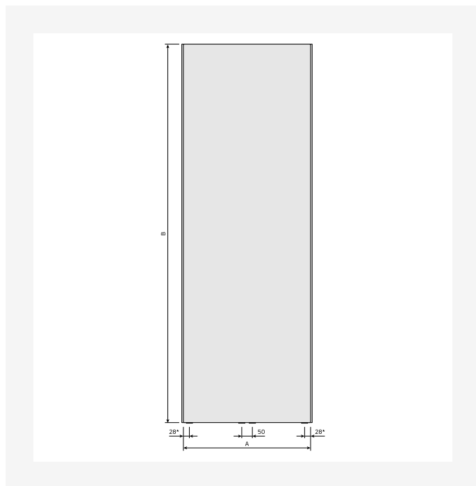
DimensionalDrawing - Kos V, eesvaade
