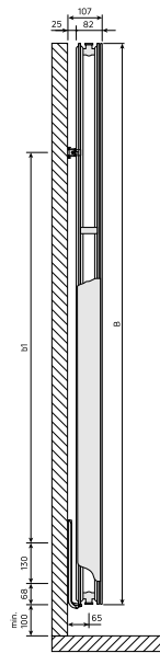
Dimensional Drawing - Kos V / Faro V, tüüp 20, külgsaade
