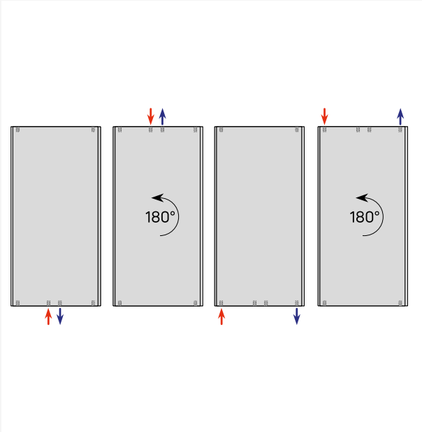
DimensionalDrawing - Vertikaalsed ühendusvariandid
