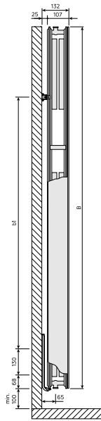
DimensionalDrawing - Kos V / Faro V, tüüp 22, külgsaade
