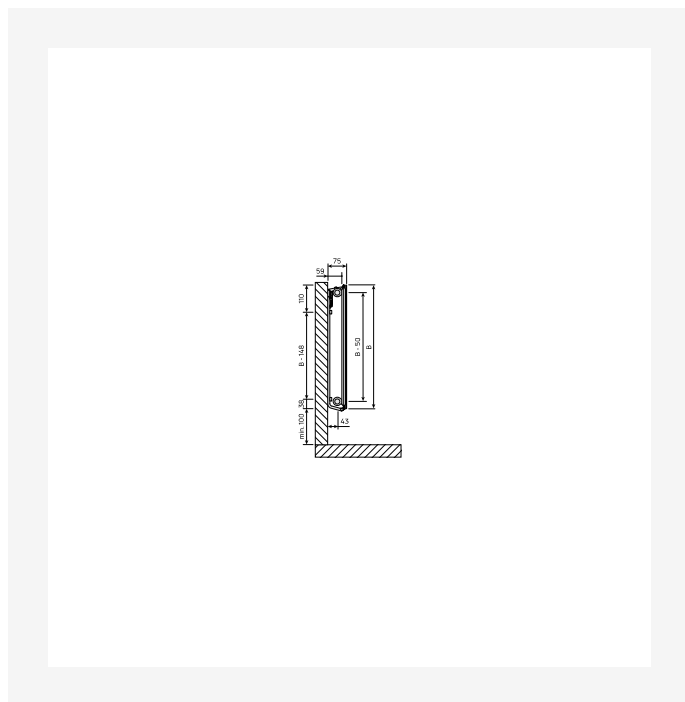
DimensionalDrawing - Plan Hygiene, tüüp 10, külgsaade, MCK
