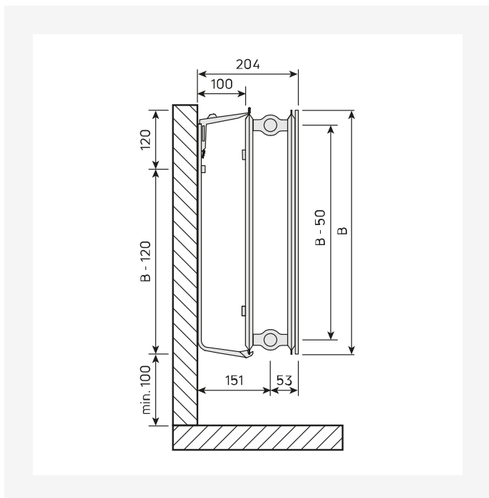
DimensionalDrawing - Plan Hygiene, tüüp 20, külgsaade
