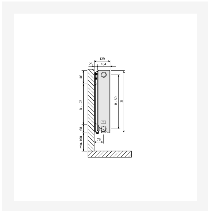
DimensionalDrawing - Ventil Compact Plan, tüüp 22, külgsaade
