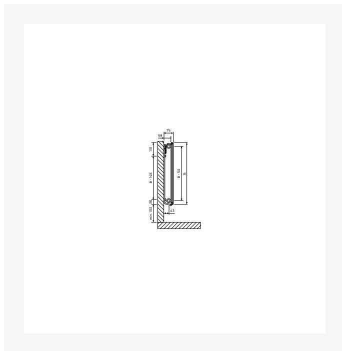
DimensionalDrawing - Plan Hygiene, tipas 10, vaizdas iš šono, MCK
