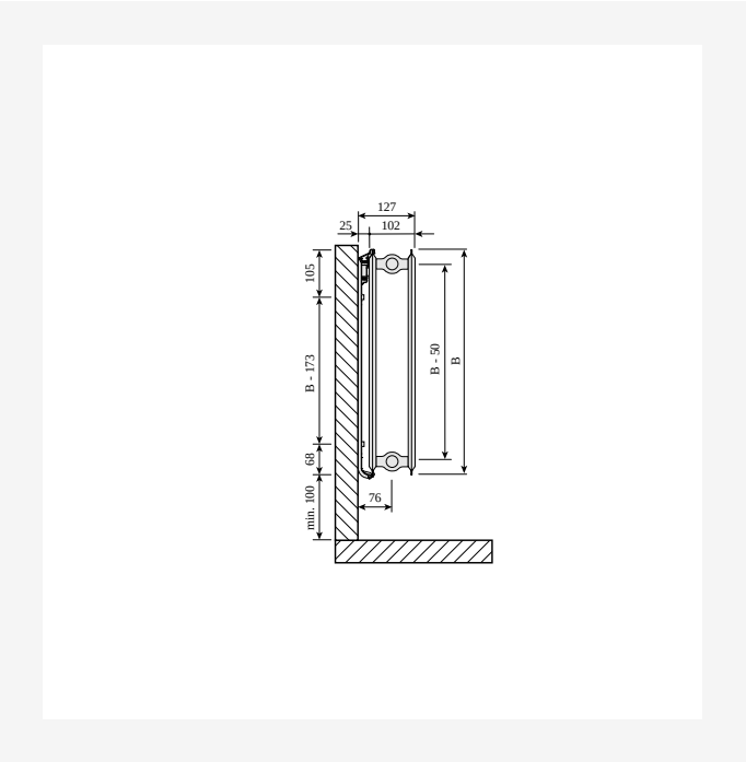
DimensionalDrawing - Hygiene, tips 20, skats no sāniem ar Monclac sienas kronšteiniem
