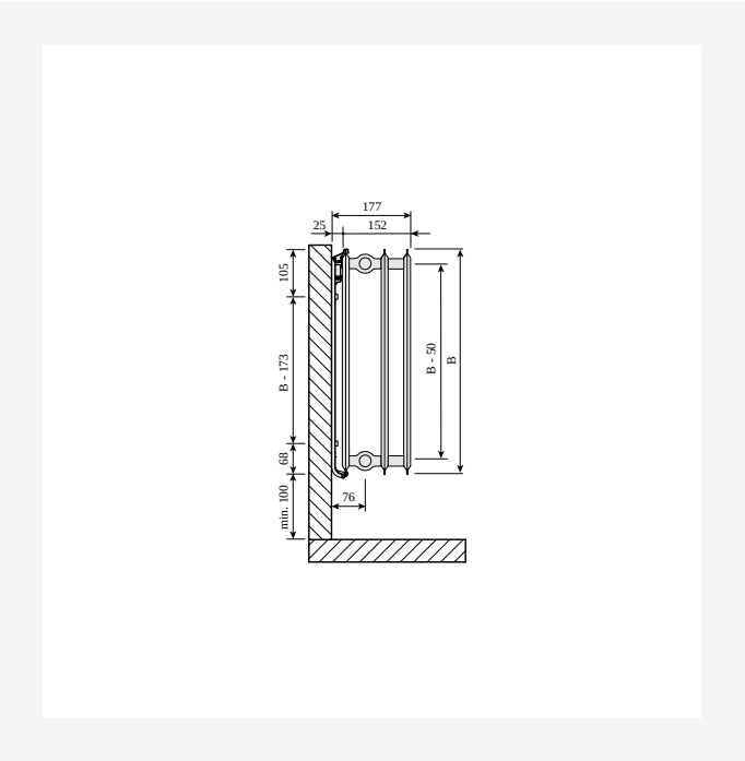
DimensionalDrawing - Hygiene, tips 30, skats no sāniem ar Monclac sienas kronšteiniem
