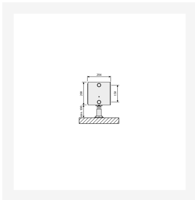
DimensionalDrawing - Plint P og Plint R, type 44, med gulvbeslag, sidevisning
