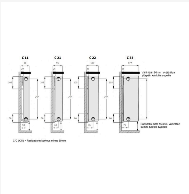
DimensionalDrawing - Monteringsvejledning til radiator
