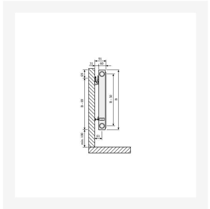
DimensionalDrawing - Compact, type 11, sidevisning med SSMS-vægbeslag
