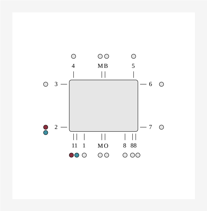
DimensionalDrawing - Botten och sidoanslutning vänster, ETIM 11
