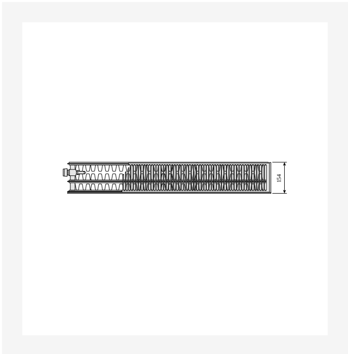
DimensionalDrawing - Thermopanel Plan typ 33, vänster toppvy
