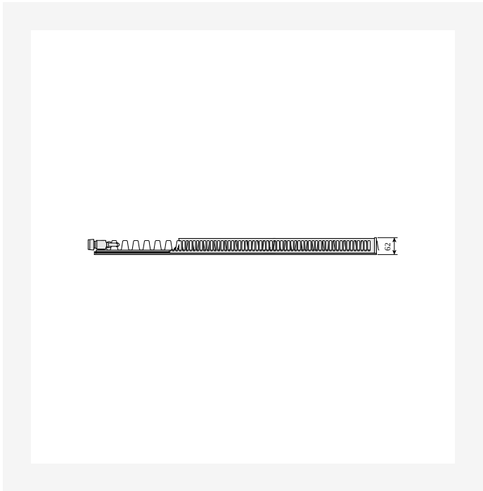
DimensionalDrawing - Thermopanel Plan typ 11, vänster toppvy
