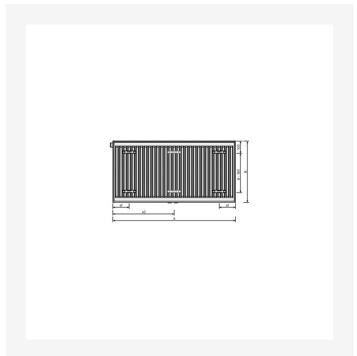
Måttitning - Flex, type 21, 22, 33, baksidesvy
