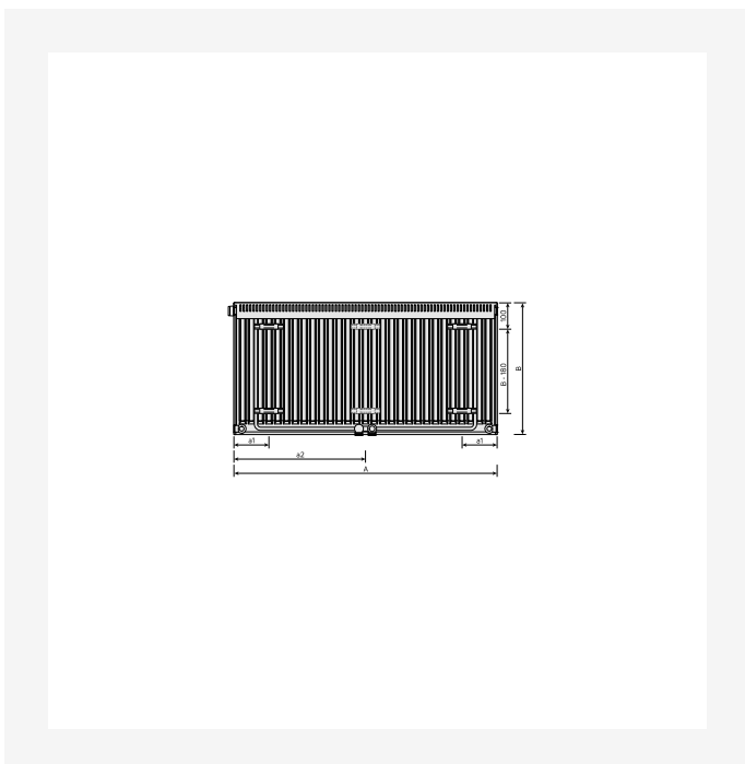
Måttitning - Flex, typ 11, baksidesvy
