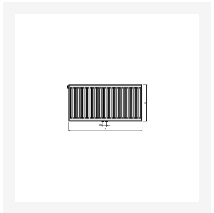
Måttitning - Plan/Ramo/Flex baksidesvy typ 21,22,33
