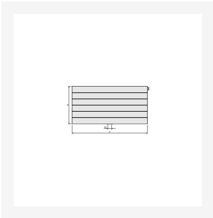
Måttitning - Ramo Flex Frontview
