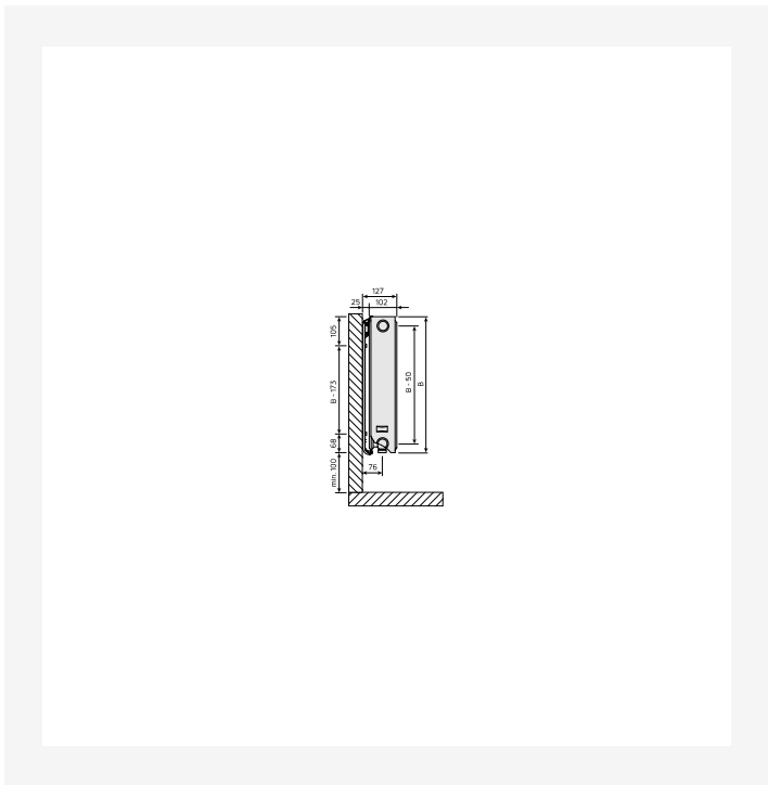
Schiță dimensională - PR-Ventil-Compact-T20-T22-SV-Monclack-3220
