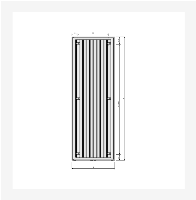
DimensionalDrawing - Tinos V, vedere din spate
