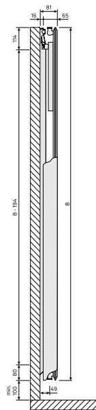
Schită dimensională - New_Tinos V-Paros V_SV_T11_0124
