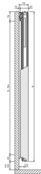
Schită dimensională - New_Tinos V-Paros V_SV_T21_0124
