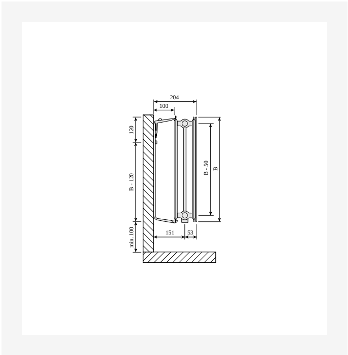
DimensionalDrawing - Plan Ventil Hygiene, tip 20, vedere laterală
