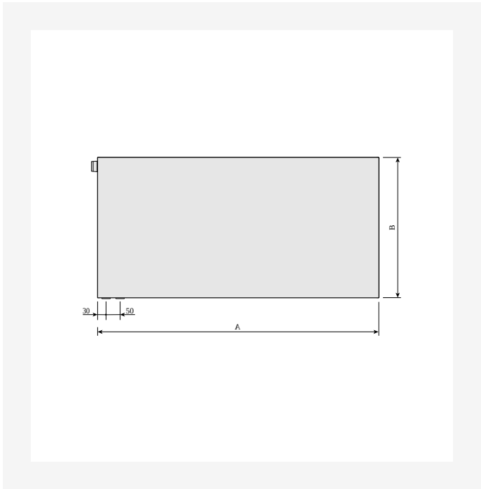
DimensionalDrawing - Plan Ventil Hygiene, vedere frontală, stânga
