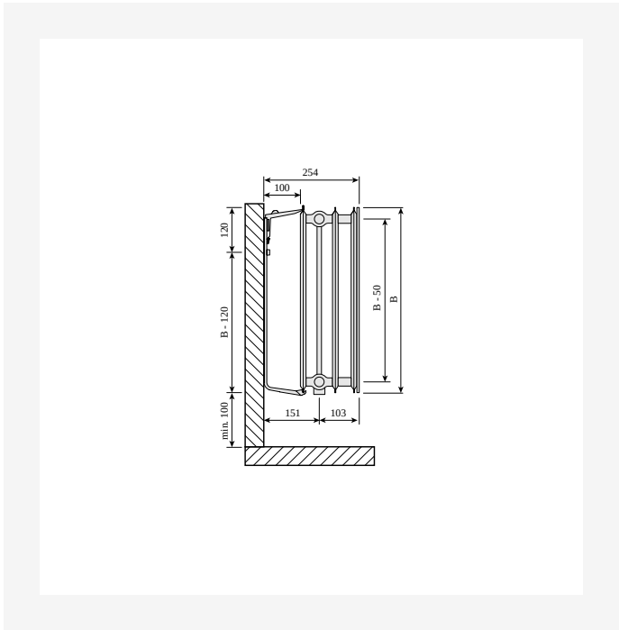
DimensionalDrawing - Plan Ventil Hygiene, tip 30, vedere laterală
