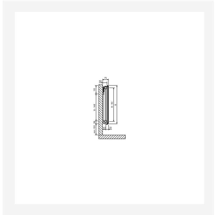
Schiță dimensională - PR-Plan-Ventil-Hygiene-T10-SV-MCK66-0121
