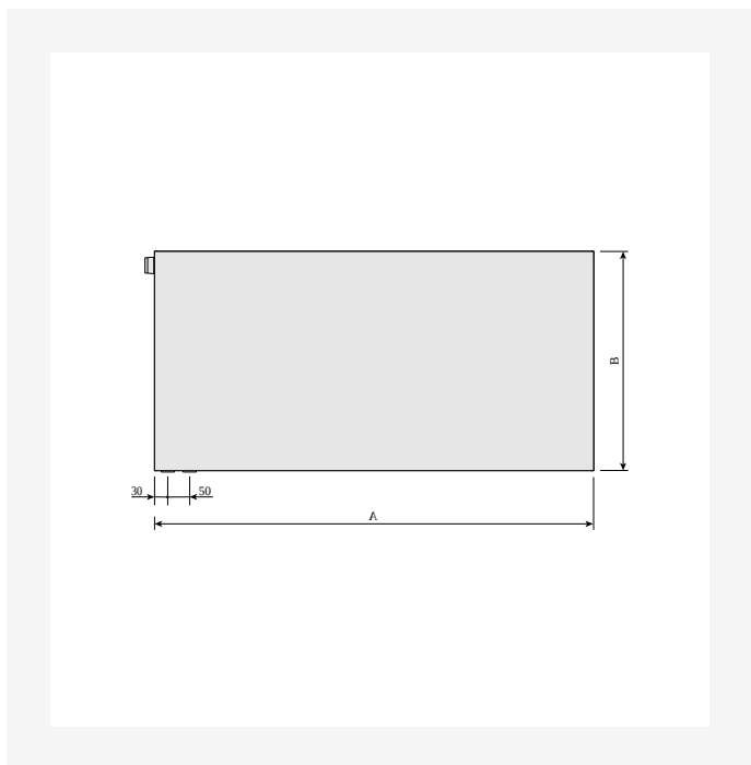
DimensionalDrawing - Plan Ventil Compact, vedere frontală stânga
