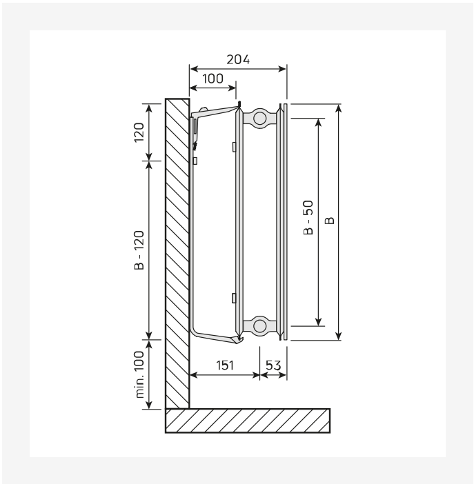
DimensionalDrawing - Plan Hygiene, tip 20, vedere laterala
