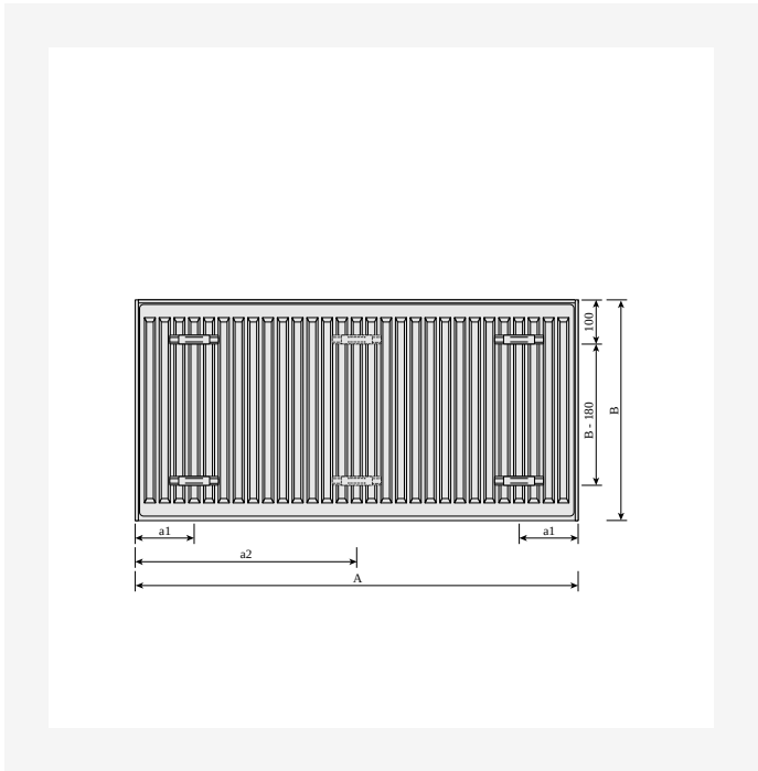
DimensionalDrawing - Compact, vedere din spate
