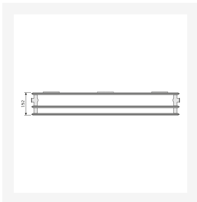
DimensionalDrawing - Hygiene, tip 30, vedere de sus
