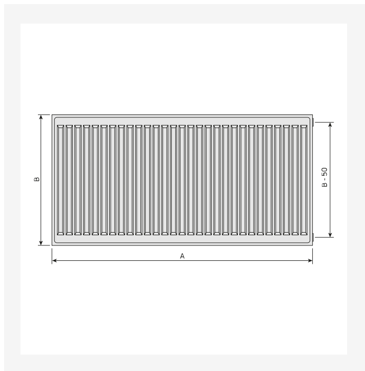
Schiță dimensională - Hygiene, vedere din fata
