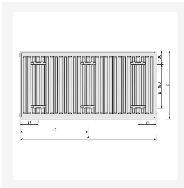
Schiță dimensională - Hygiene, vedere din spate
