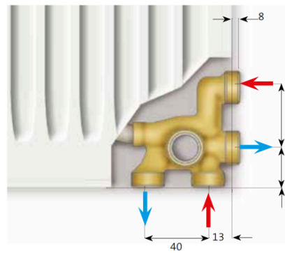
V4 BOTTEN OCH SIDA 2-RÖR
