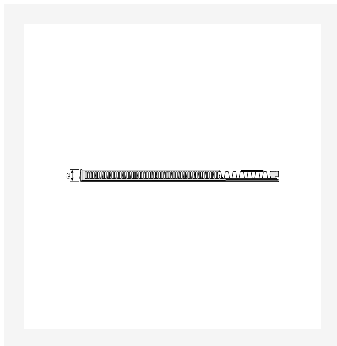
DimensionalDrawing - Ramo Compact, tipas 11, vaizdas iš viršaus
