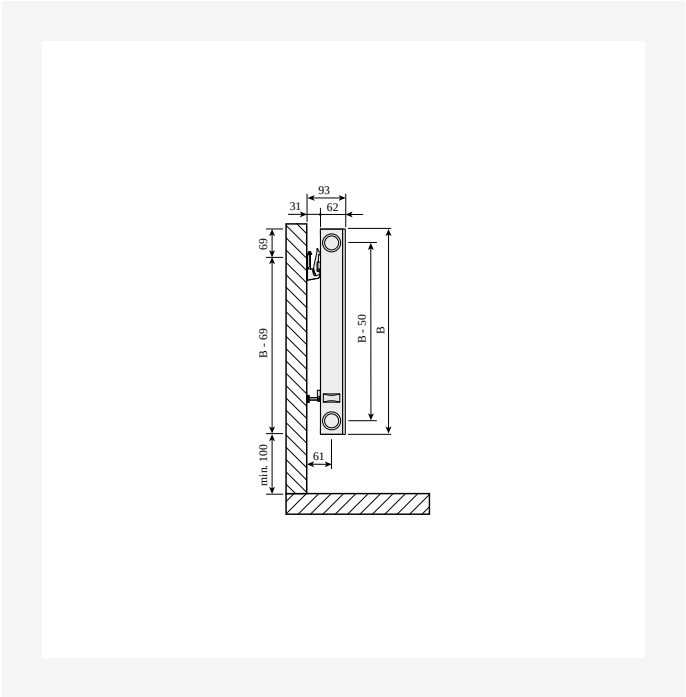
DimensionalDrawing - Ramo Compact, tipas 11, vaizdas iš šono su SSMS sieniniais laikikliais
