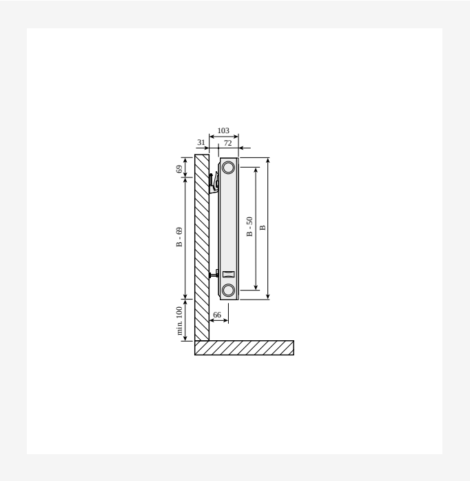
DimensionalDrawing - Ramo Compact, tipas 21s, vaizdas iš šono su SSMS sieniniais laikikliais
