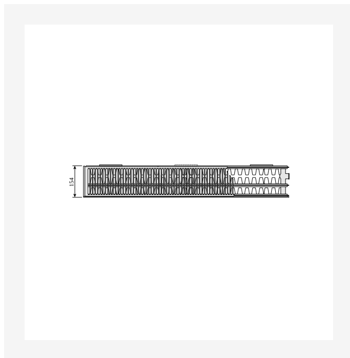
DimensionalDrawing - Ramo Compact, tipas 33, vaizdas iš viršaus
