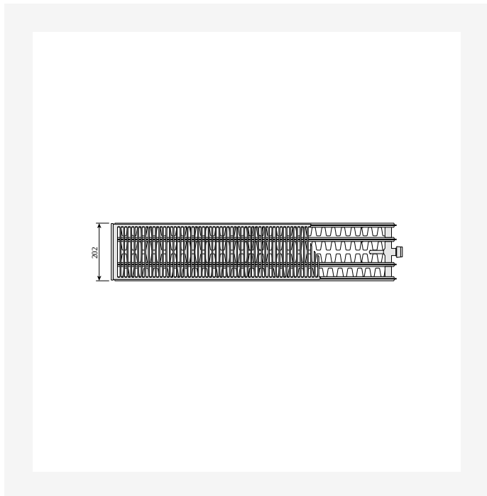
DimensionalDrawing - Plint, tipas 44, vaizdas iš viršaus
