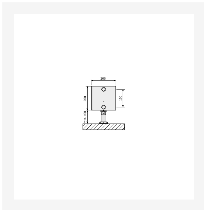
DimensionalDrawing - Plint PD ir Plint RD, tipas 44, su grindų laikikliais, vaizdas iš šono
