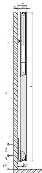
DimensionalDrawing - Kos V / Faro V, tipas 21, vaizdas iš šono
