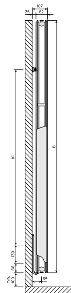
DimensionalDrawing - Kos V / Faro V, tipas 20, vaizdas iš šono
